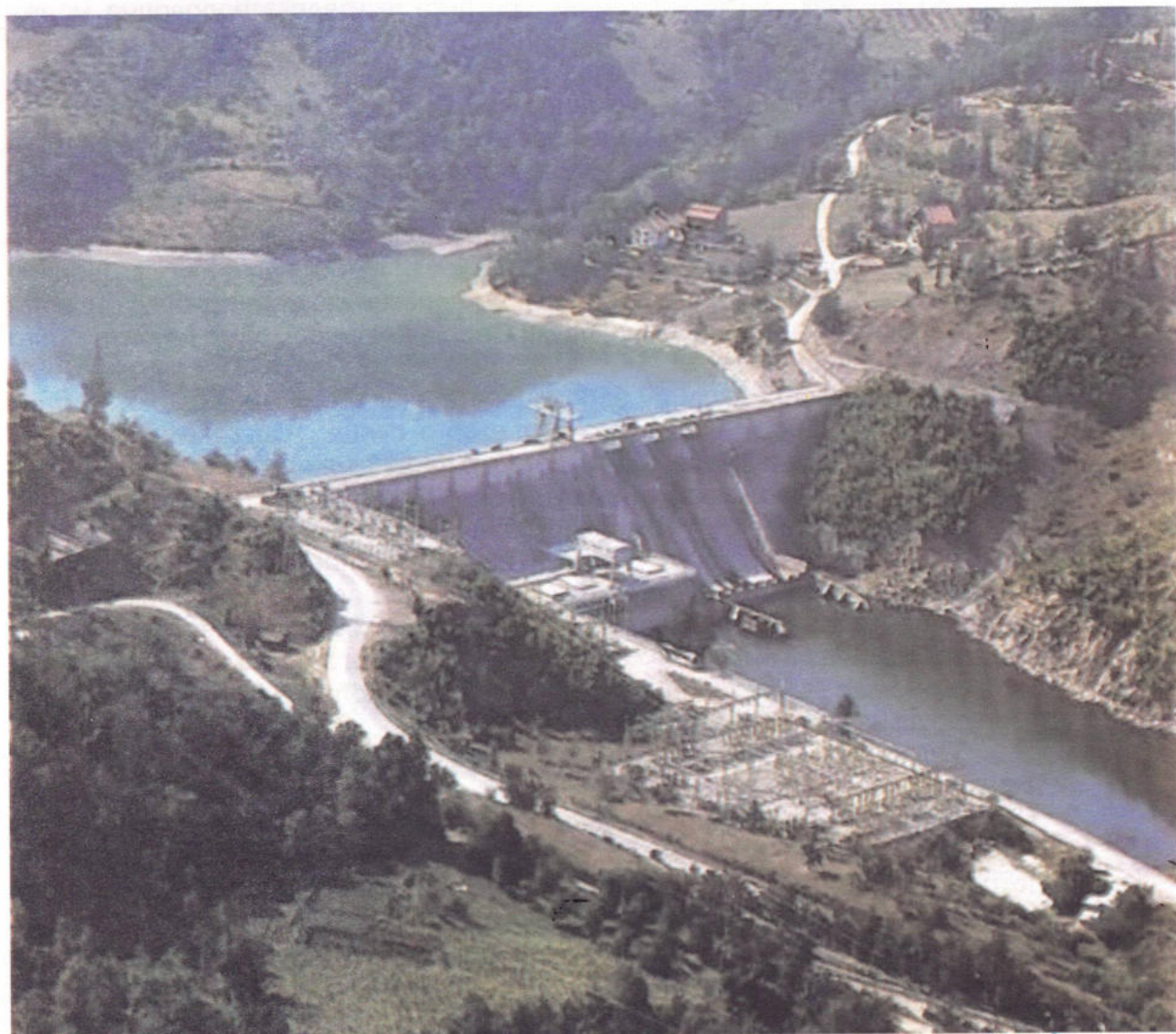
Брана, машинско постројење и део акумулационог језера ХЕ Потпећ
